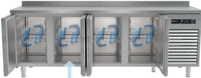
Sökülüp Takılabilen, Geçmeli Özel Tasarım Tel Raf Dikmeler Dismountable shelf holder attachments
